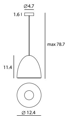
Castle Pendant M SQ-7132CP E26 1 x Max 100W Materials : concrete, steel
