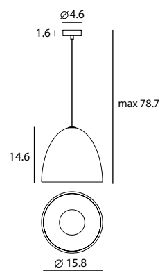
Castle Pendant L SQ-7133CP E26 1 x Max 77W Materials : concrete, steel
