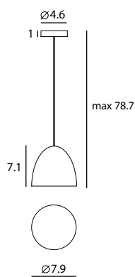
Castle Pendant S SQ-7131CP E26 1 x Max 100W Materials : concrete, steel
