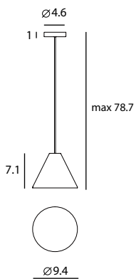
Castle Pendant Cone SQ-185CP E26 1 x Max 77W Materials : concrete, steel
