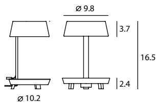
Carry Table Mini SQ-6353MDU E26 1 x Max 60W on/off rocker switch Materials : steel, beech Color : matte black & red / matte white & beech USB charger
